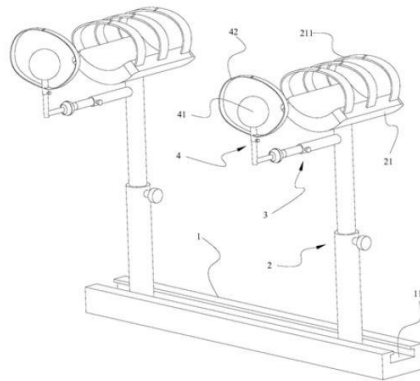
Resim 6. Piyanoda Öğretimi için Yardımcı Cihaz'ın çizimleri (Lei, Yu ve Committee, 2018).
