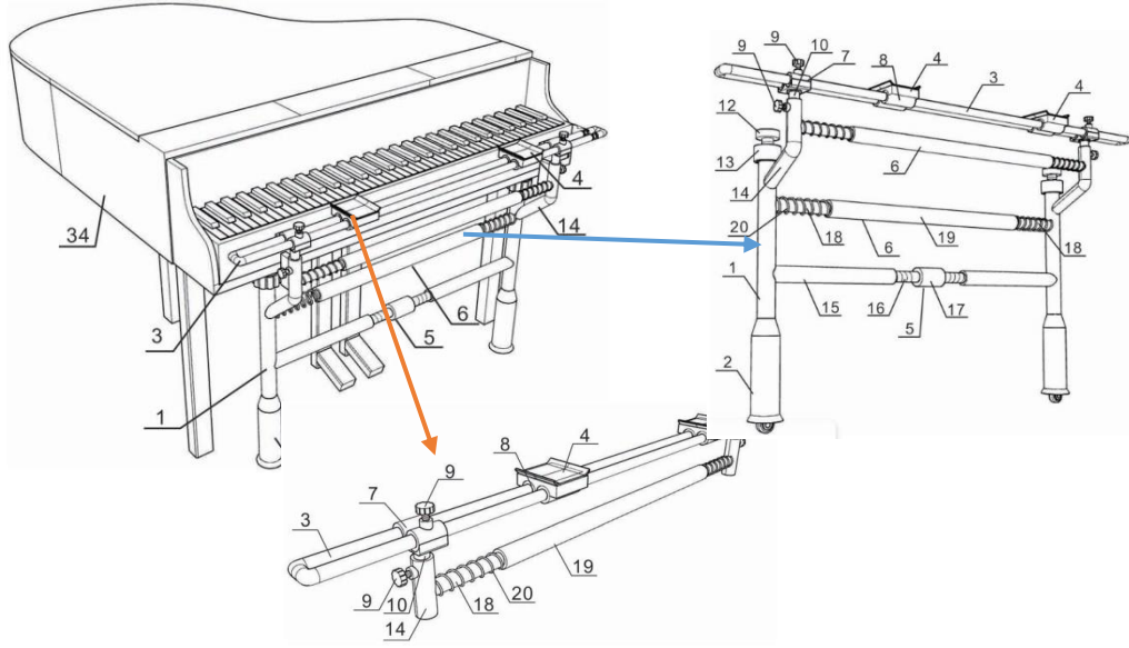
Resim 5. Piyanoda Çalışmasına Yardımcı Olan Bir Tür El Tipi Doğrultucu'nun çizimleri (Bo ve Yu, 2018).
