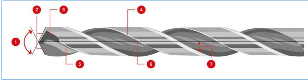
Şekil 4. Matkap ucu geometrisi ve tanımlamaları (URL 1).
